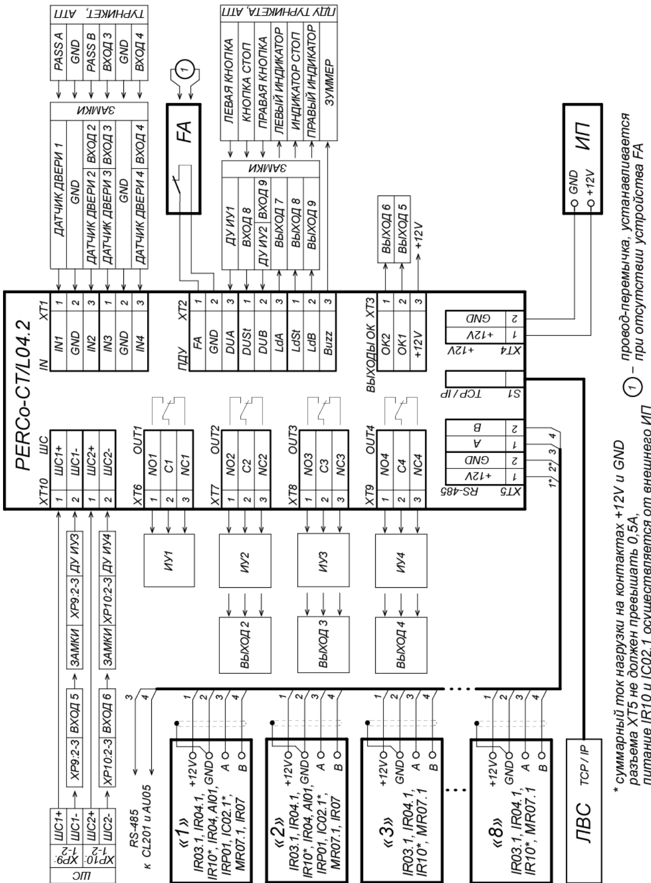
Рисунок 3. Общая схема подключений
