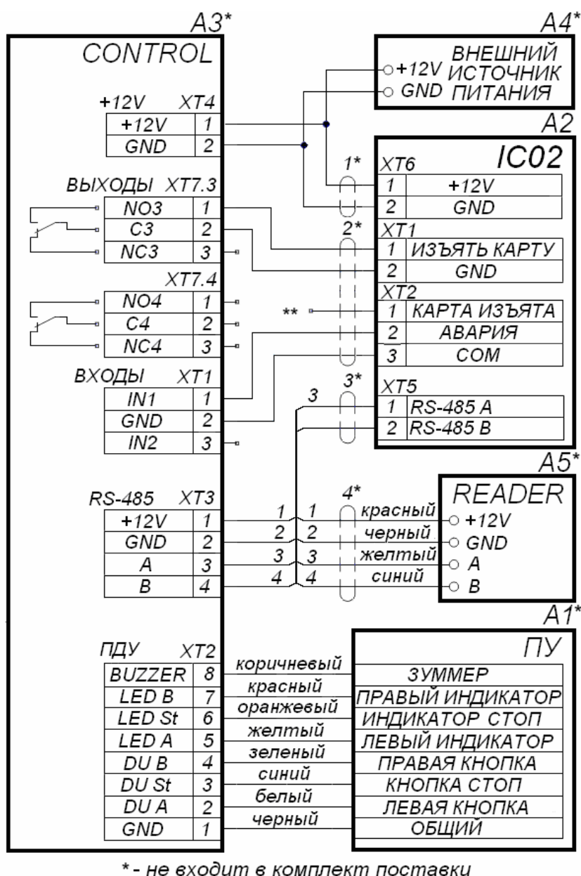
Рисунок 7 Схема подключения картоприемника к контроллеру PERCo-CT/L04 1
