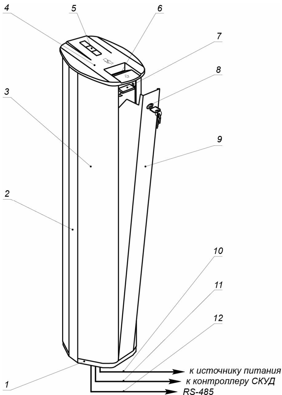
Рисунок 2 Устройство картоприемника:
