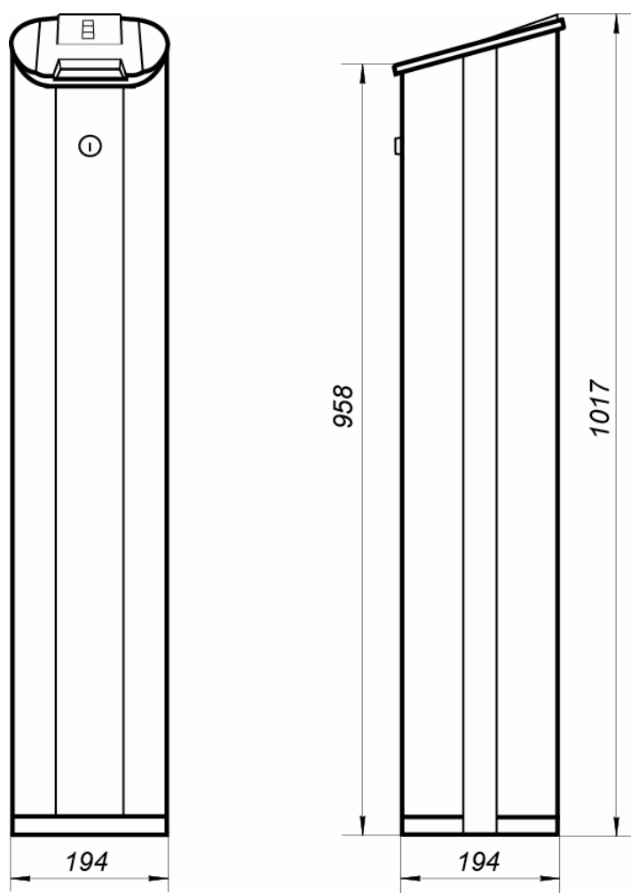
Рисунок 1 Габаритные размеры картоприемника
