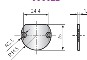
Монтажная пластина для замка EP303
