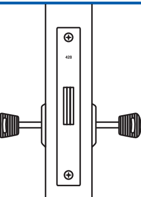
Замок для деревянных и металлических дверей.
