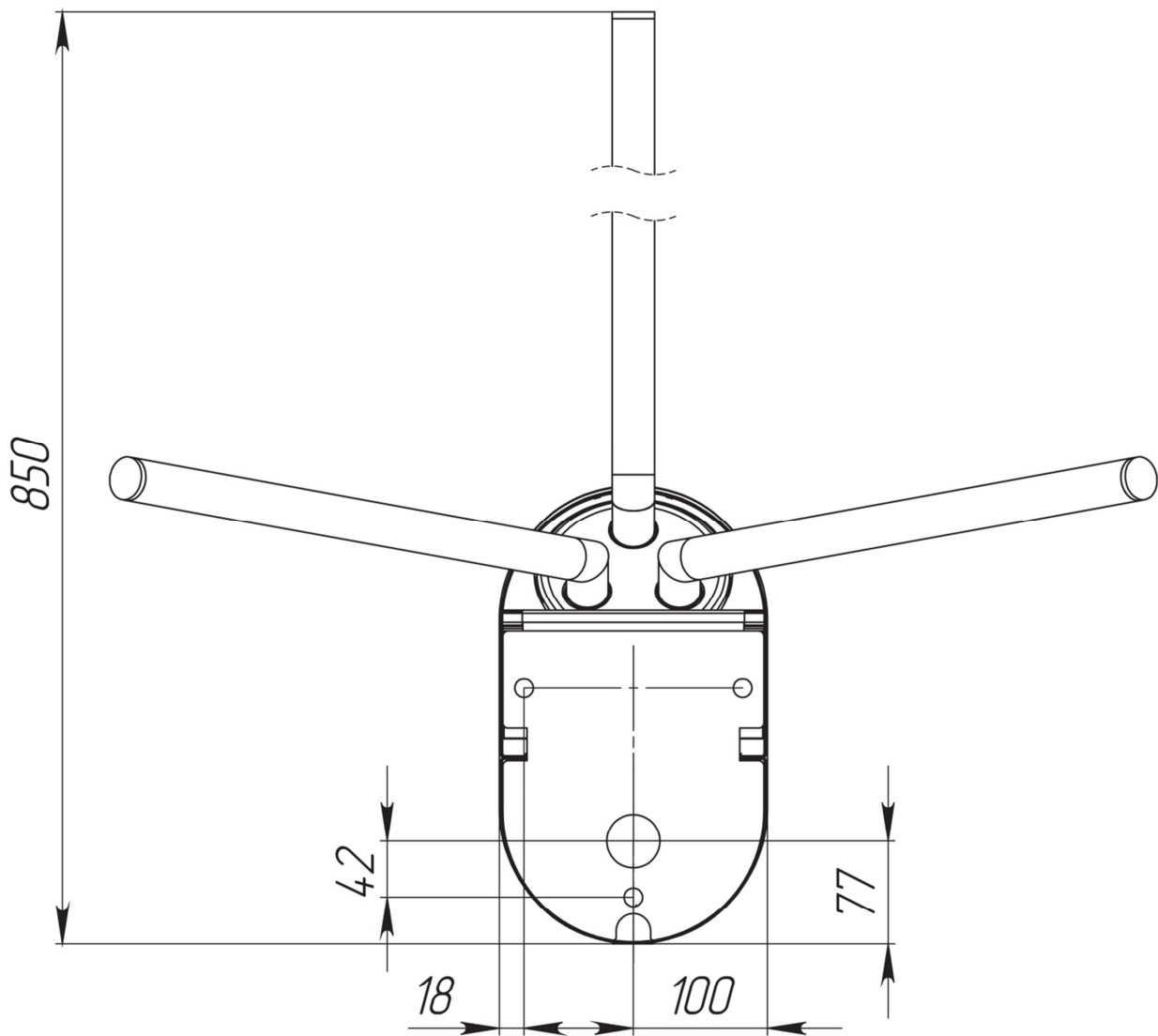
Рис. 11. Расположение монтажных отверстий относительно внешних габаритов турник
