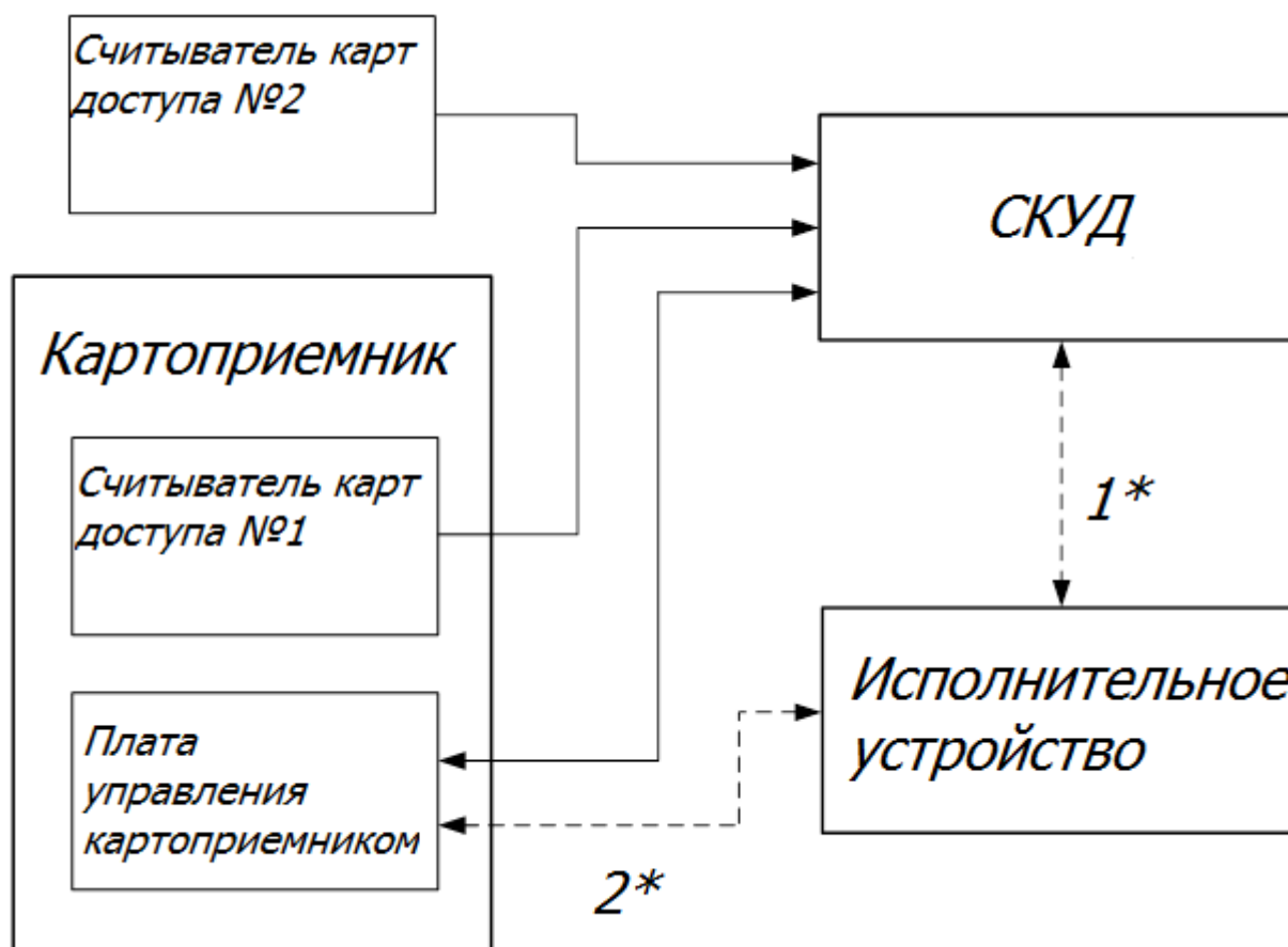
Рис. 10. . Структурная схема №1
