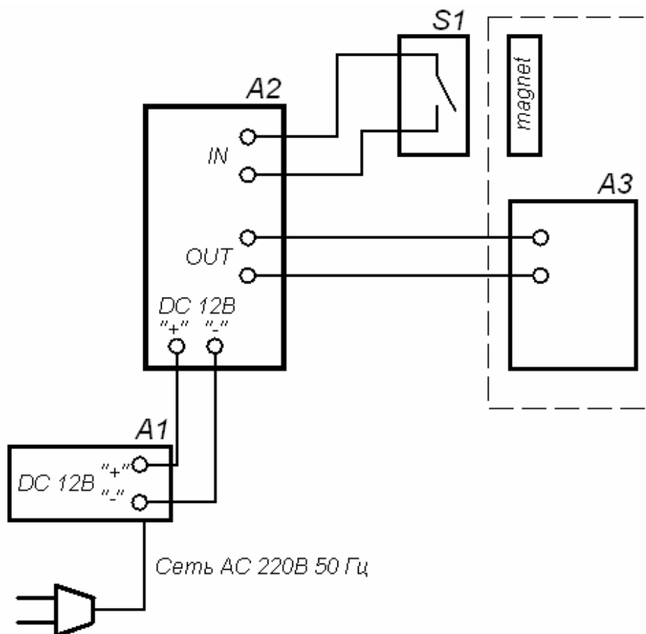
Рисунок 2. Схема подключения замка
