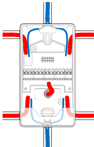
Рис 10. Подвод кабелей
