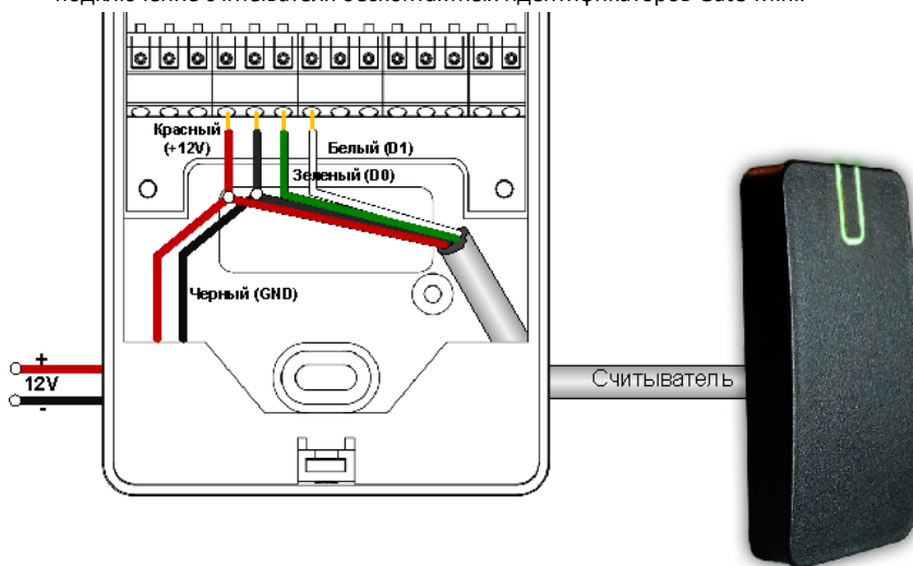
Рис.13. Подключение внешнего считывателя
