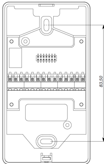
Рис 11. Задняя пластина
