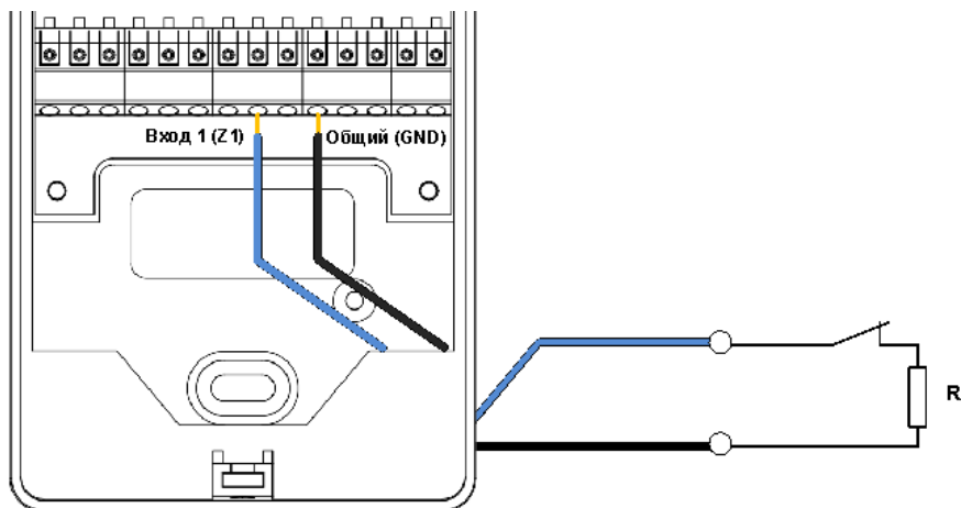
Рис.15. Подключение дверного контакта
