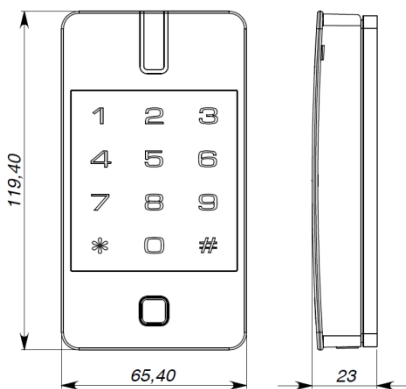
Рис 9. Габаритные размеры
