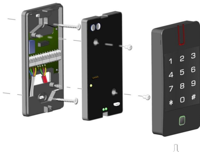
Рис 12. Установка контроллера
