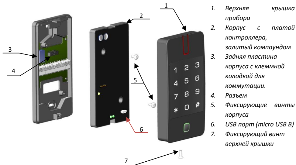
Рис. 2. Внешний вид компонентов Gate-IP-Combo модификации 2
