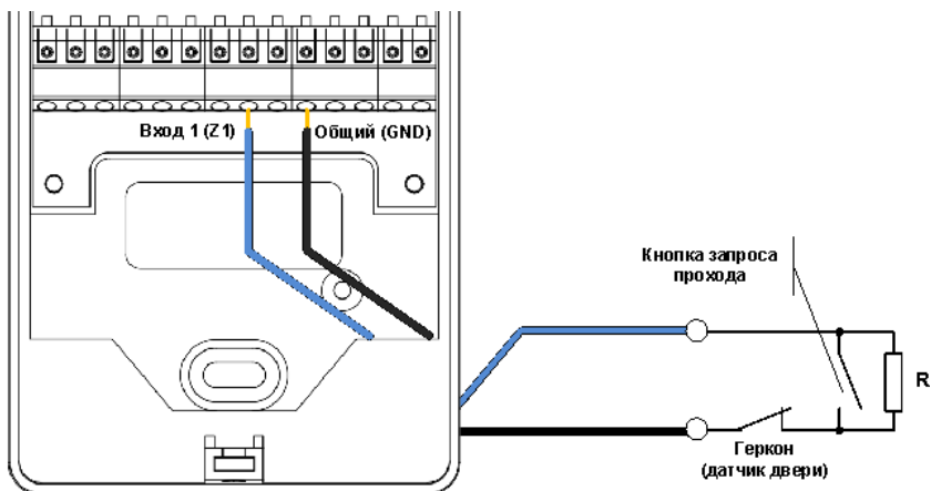
Рис.16. Подключение комбинированного шлейфа
