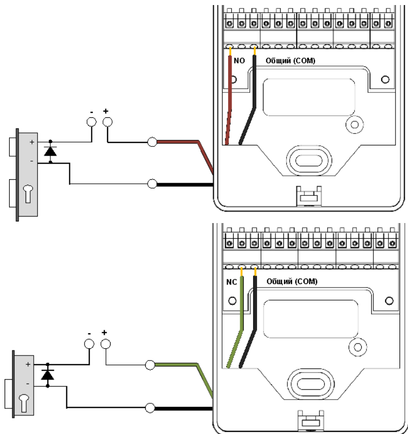
Рис.18. Подключение замков
