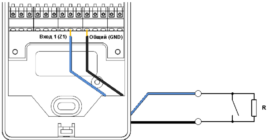
Рис.14. Подключение кнопки запроса прохода
